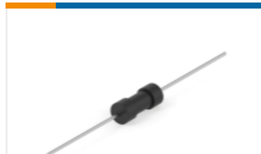
TE Part # 3-2176471-3 HPCR 0819 A 10% 470R Std T&R HV
