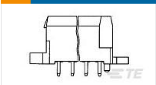
TE Part # 963357-2 2X 9P MESSERLEISTE
