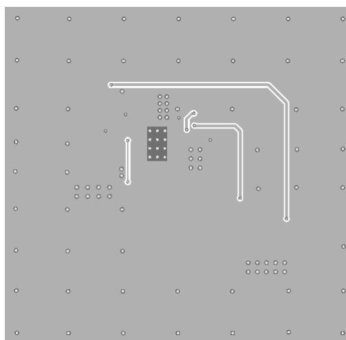
Inner Layer 2
