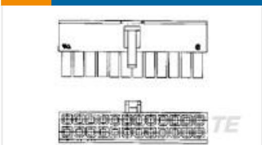
TE Part # 1-1586765-0 10P RCPT VAL-U-LOK GW
