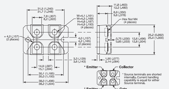
SOT-227
