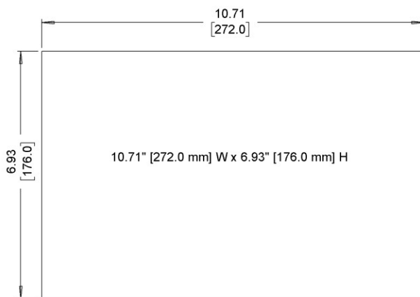
Cutout Dimensions
