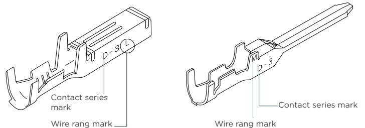
Receptacle Contact
