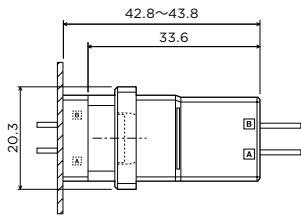
Panel /Free Hanging type
