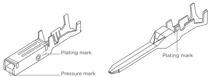
Receptacle Contact
