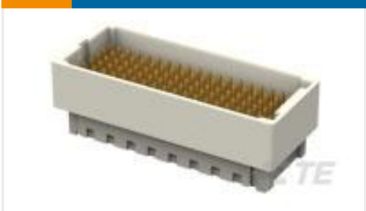
TE Part # 2102060-4 Mezalok, Pin, 114 p, 30 Au, LF
