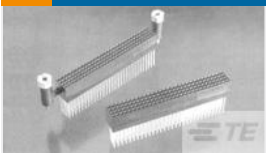
TE Part # 1375800-3 ASSY, 120 POS PC104 PLUS
