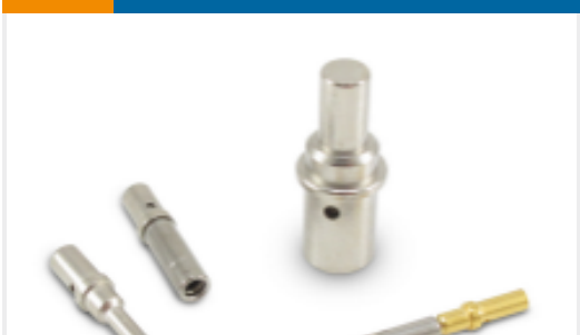
TE Part # 0462-201-20141 DEUTSCH Solid Contacts
