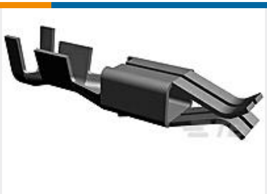
TE Part # 925590-4 MINI SPRING REC.
