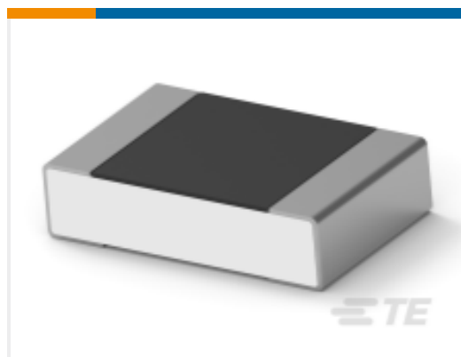
TE Part # 4-2176375-9 RQ 0805 3K65 0.1% 10PPM 1K RL
