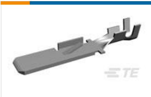
TE Part # 969031-2 POS-MATE FLA-STE5,2
