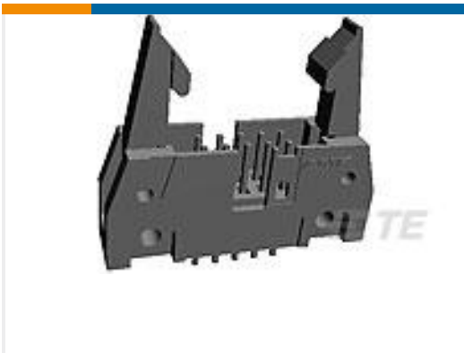
TE Part # 5499206-1 A/L UNIV HDR 10P VERT LG LAT
