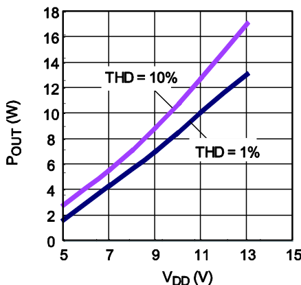
VDD vs. POUT 4Ω + 33μH
