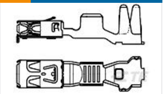
TE Part # 1411593-1 ELOP2,8 F6000Y 63
