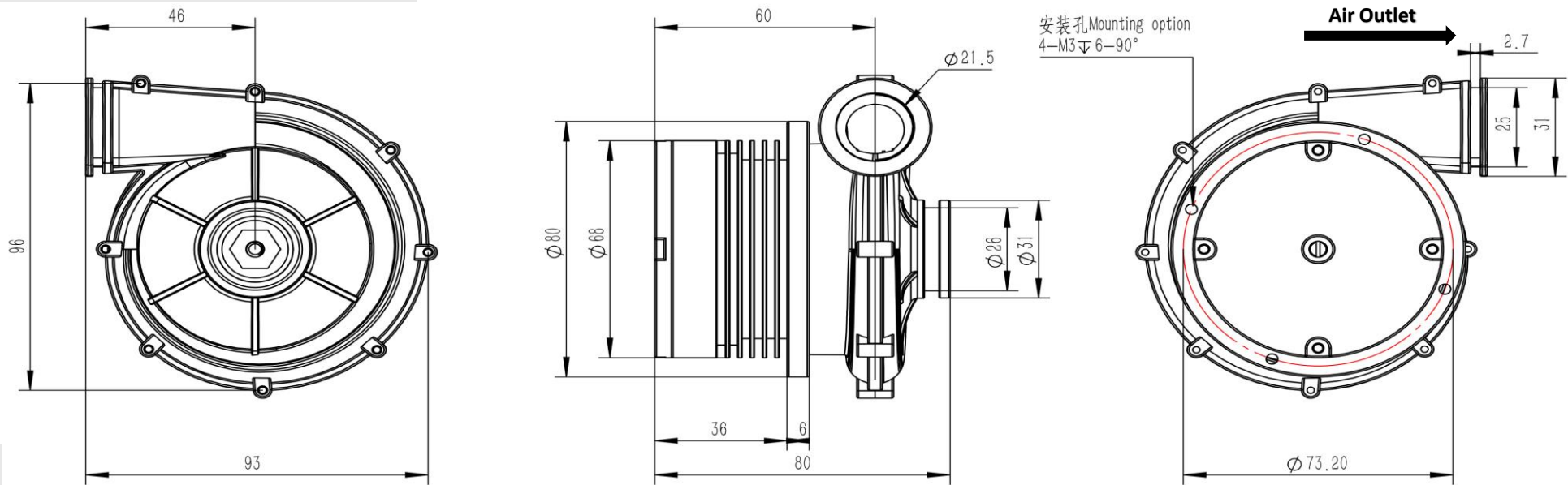
尺寸图 (OUTLINE DRAWING)
