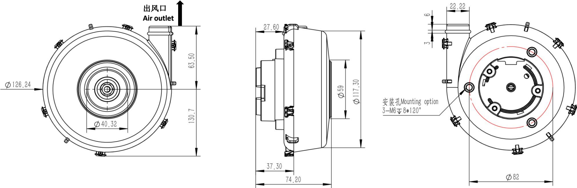
尺寸图 (OUTLINE DRAWING)
