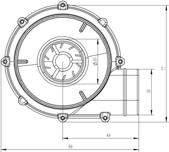
尺寸图 (OUTLINE DRAWING)
