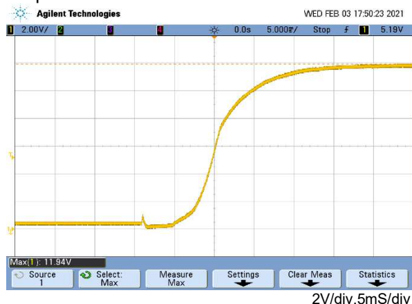
Output turn-on
