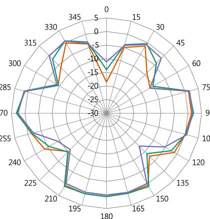
YZ-Plane Gain
