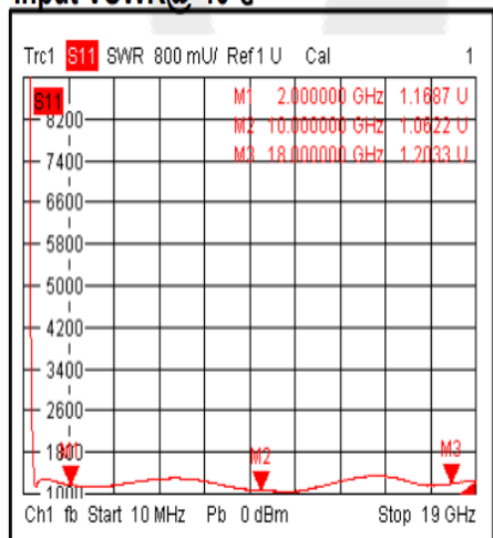
Input VSWR@-40°C
