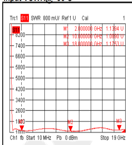
Input VSWR@+85°C
