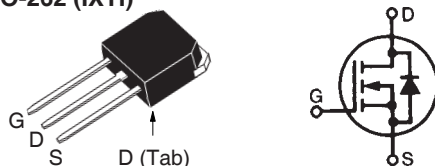
TO-262 (IXTI)
