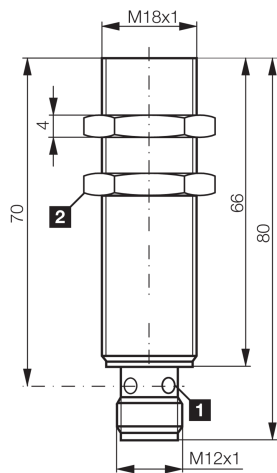
2) Schlüsselweite 24 mm
