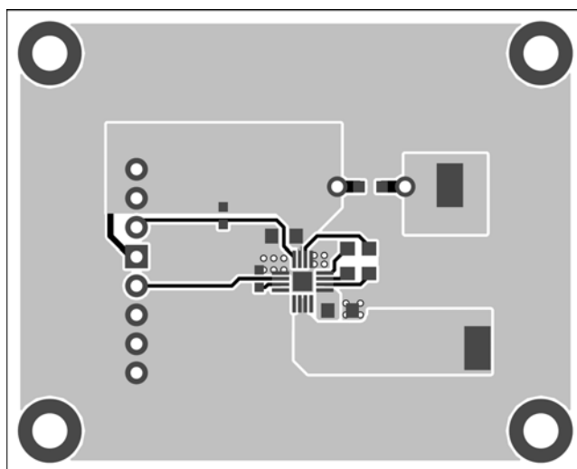
Figure 2—Top Layer
