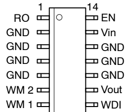
SOIC-14
