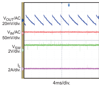
Input/Output Ripple
