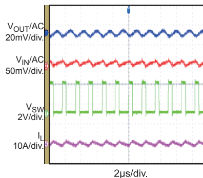
Input/Output Ripple
