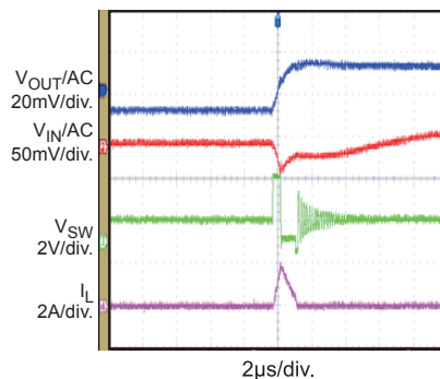
Input/Output Ripple
