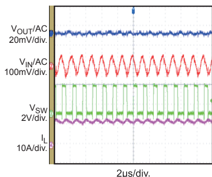
Input/Output Ripple
