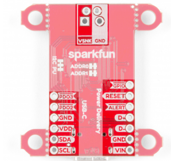
IO Pins
