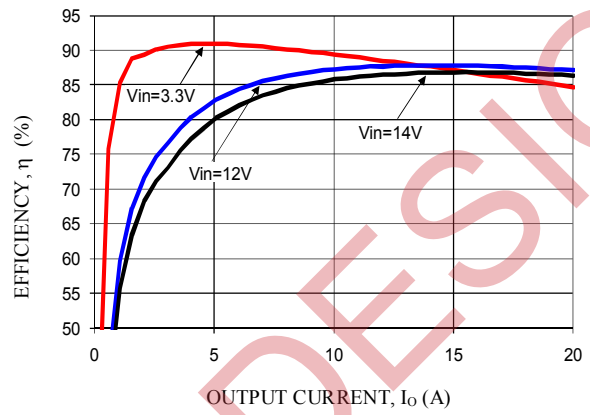
V_o=1.2V
