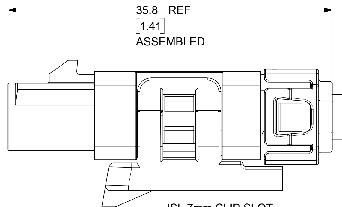
ISL 7mm CLIP SLOT
