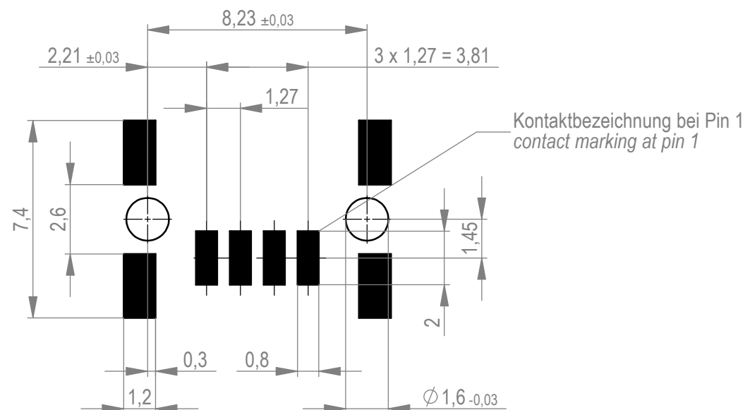
Leiterplatten-Layout für SMT PCB-Layout for SMT
