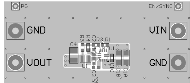
Top Layer
