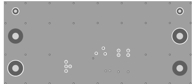
Inner Layer 1
