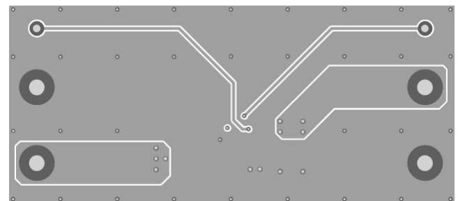
Inner Layer 2
