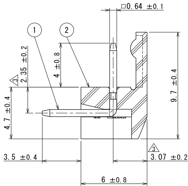
断面図 A-A
