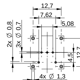
P.C.B Layout
