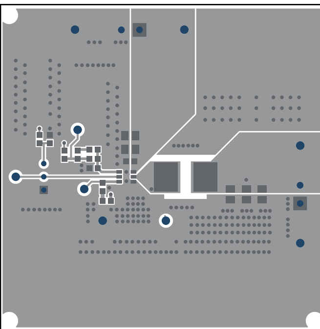
Figure 6-2. Top Layer
