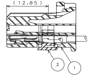
SECT. A-A (SCALE 2:1)
