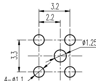
安装孔 PIERCING PLAN
