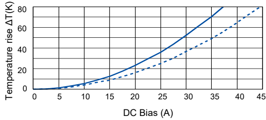
[ ETQP5MR68YLC ]
