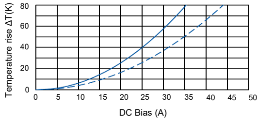
[ ETQP5MR68YLC ]
