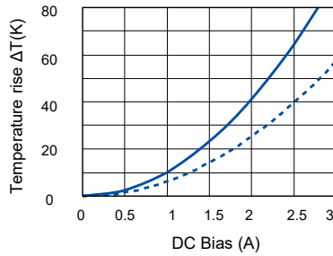
[ ETQP4M330YFN ]
