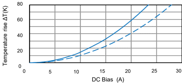
[ ETQP5M2R0YSC ]
