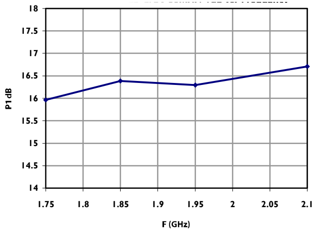
P1dB
