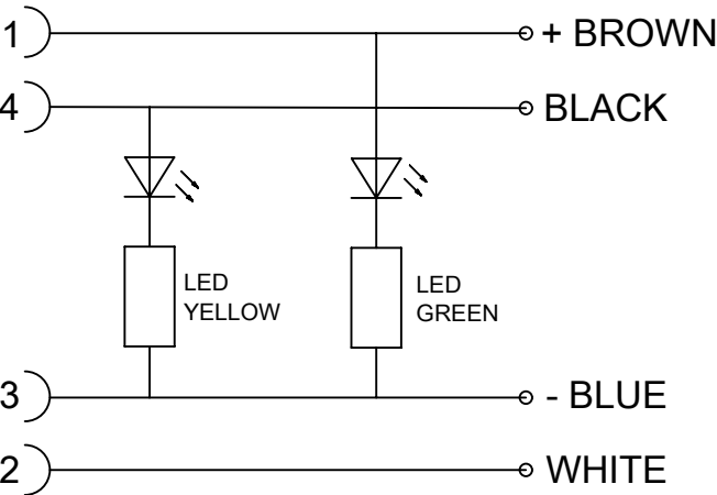
PNP WIRING
