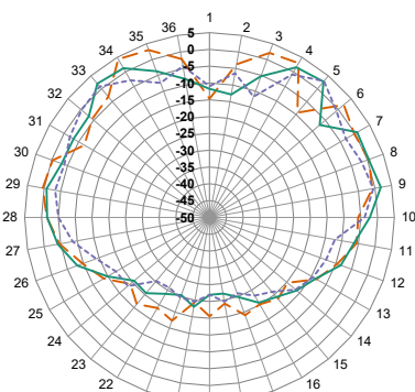
XZ-Plane Gain
