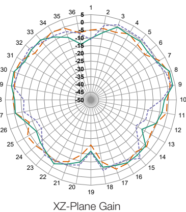
XZ-Plane Gain
