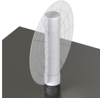
YZ-Plane Gain
