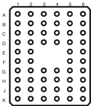
56-Ball BGA
