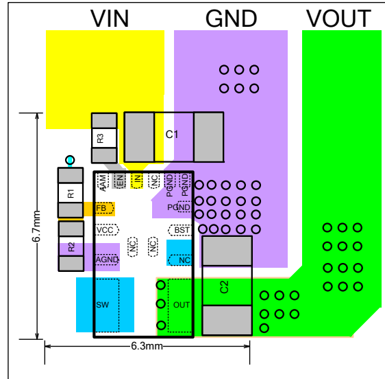
Top Layer
