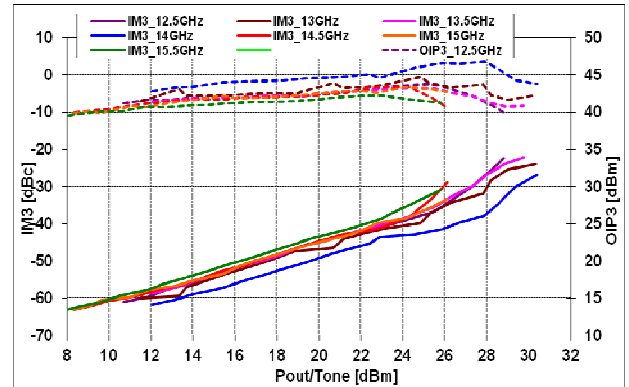
@ V_{ds}=6V , I_{ds}=2000mA
