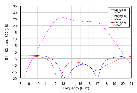
V_{ds}=5V, I_{ds}=1400mA
