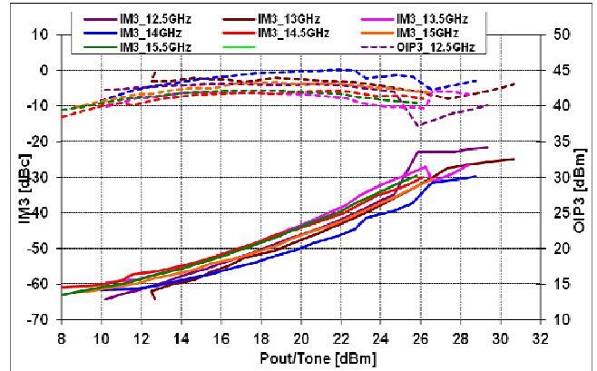
@ V_{ds}=6V , I_{ds}=1400mA
