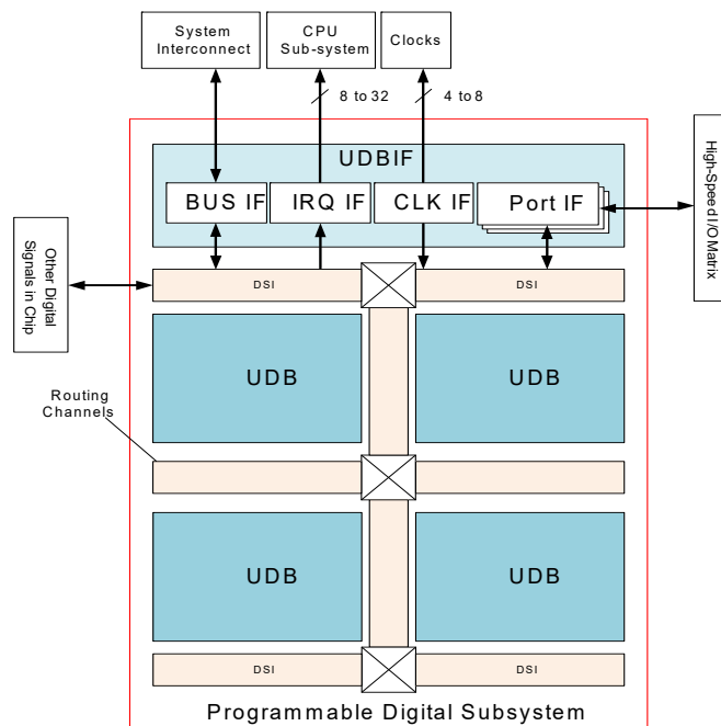
Figure 5 UDB Array
