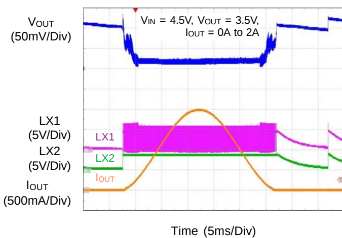
VOUT Ripple Voltage
