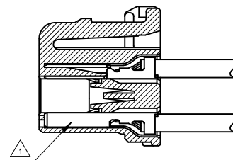
ターミナル装着図 TERMINAL ASSEMBLY DRAWING
