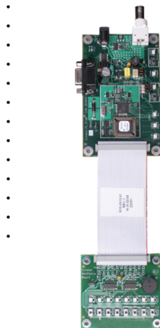
PL 3150 EVB and MiniGizmo
