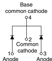
VS-30CTH02HN3
