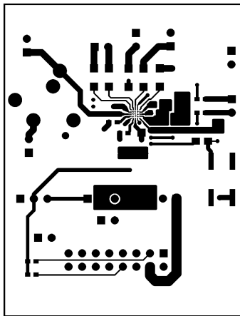
Figure 45. Top Layer
